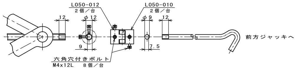
ジャッキ連結棒取付要領図
